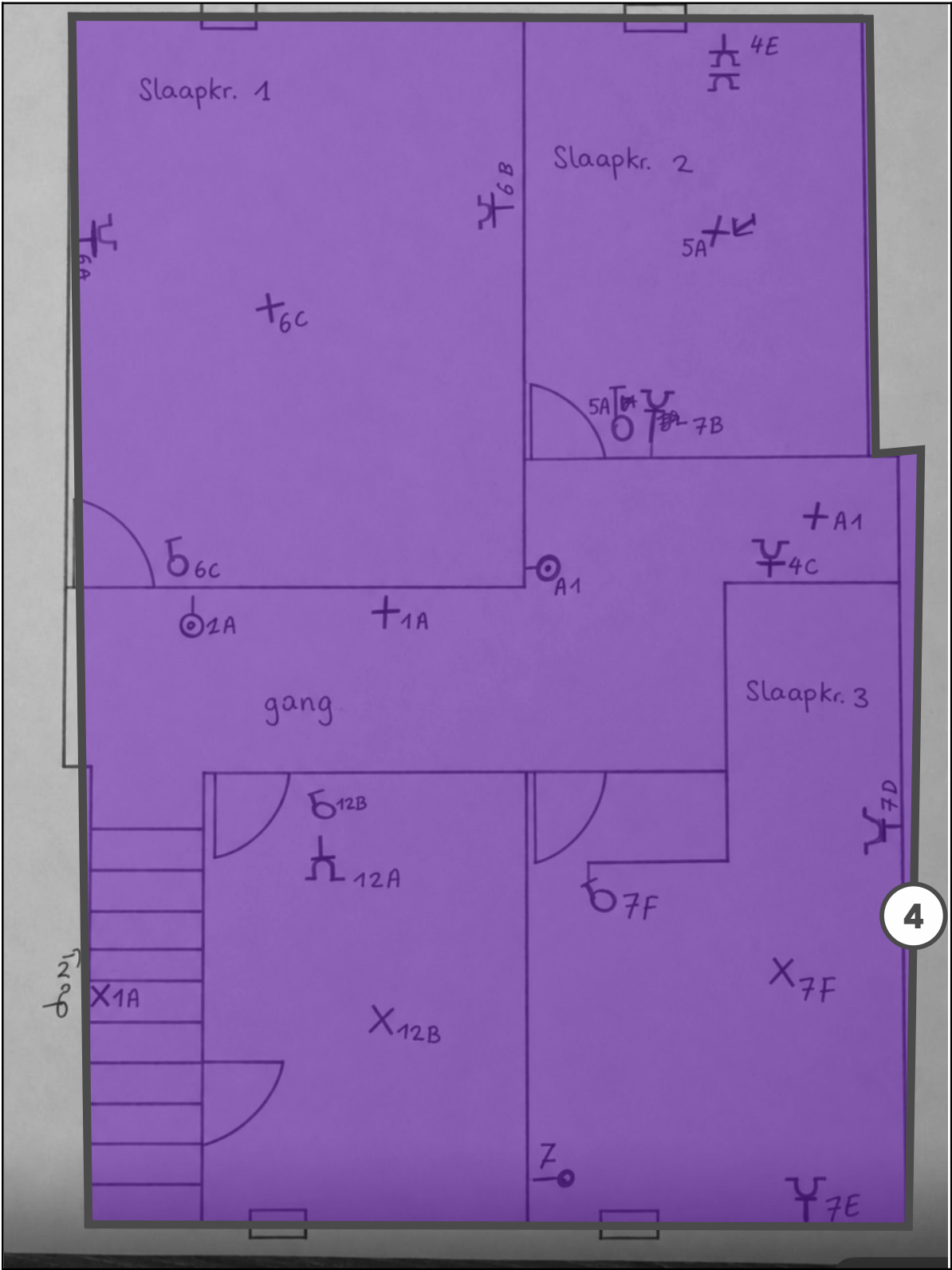
Legende van plan 1.5: Plan V+1 plafonds
