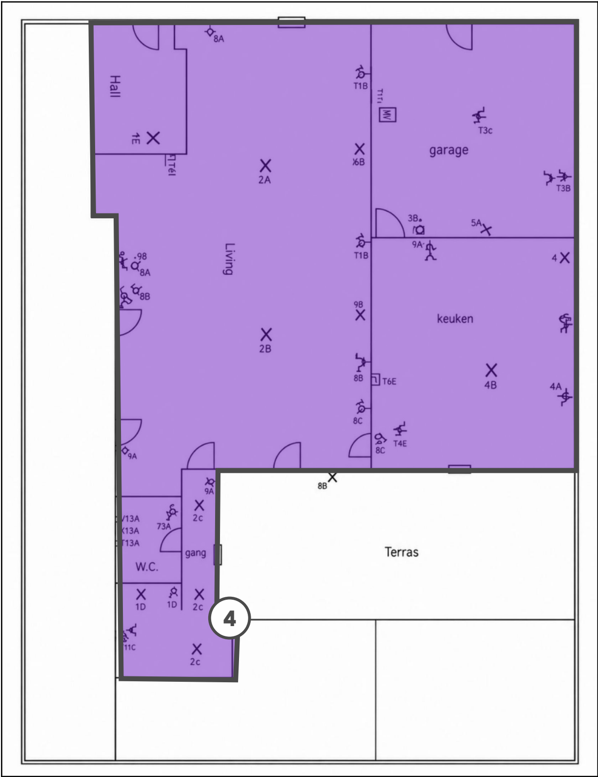
Legende van plan 1.2: Plan Gelijkvloers plafonds
